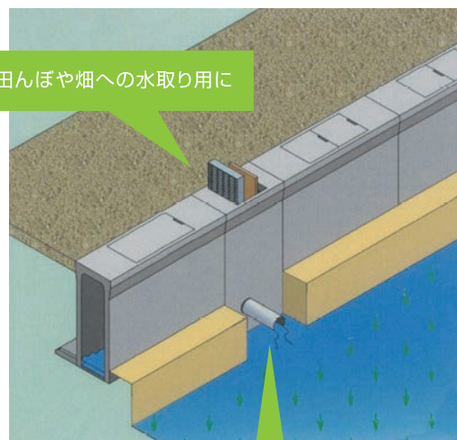
施工イメージ図
