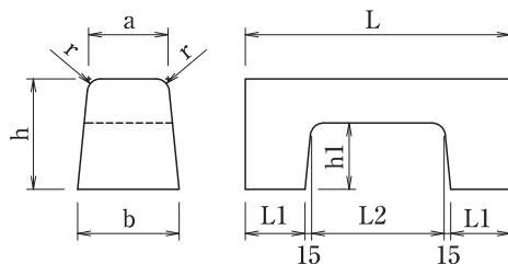
歩車道境界ブロック 両面 柵用
