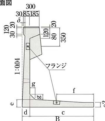
B-B矢視
