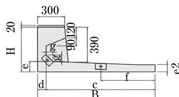
側面図
