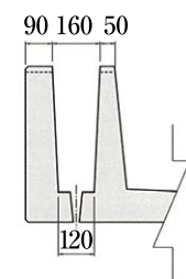
A-A矢視
