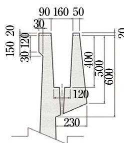
B-B矢視
