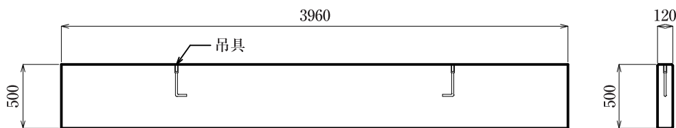
土留板 3960×500×120
