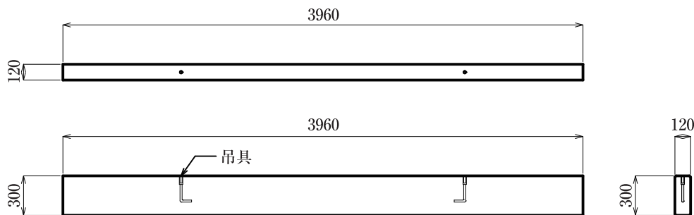
土留板 3960×300×120
