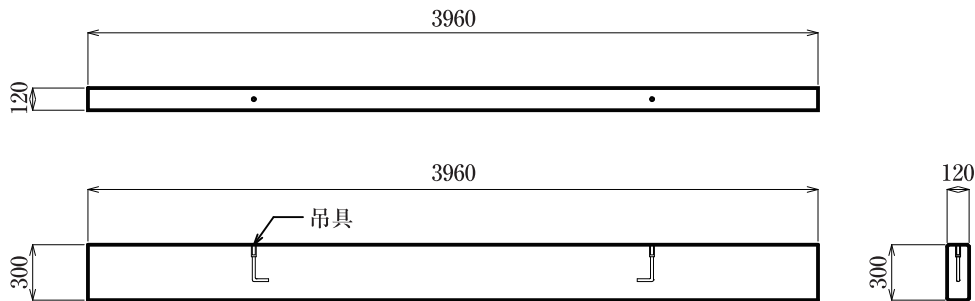
土留板 3960×300×120
