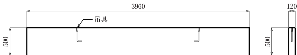
土留板 3960×500×120
