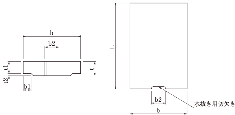
上ぶた式U形側溝蓋 PC1・PC2
