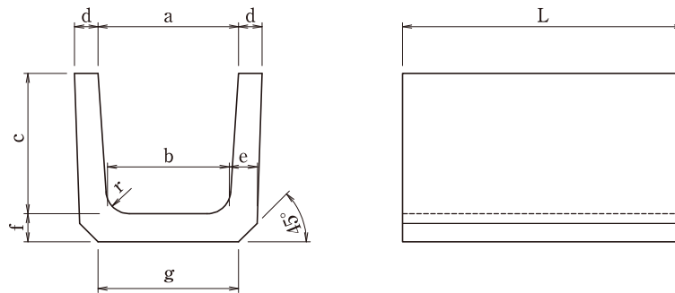
上ぶた式U形側溝 PU1
