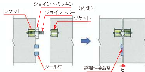
コーキングガンにより接着剤を内目地に充填
