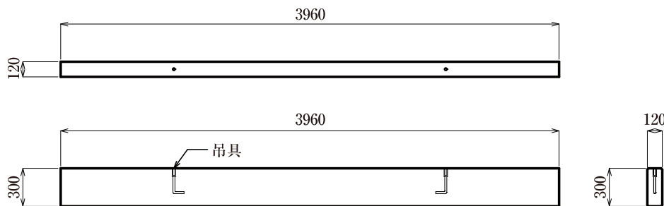
土留板 3960×300×120
