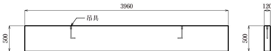
土留板 3960×500×120
