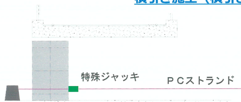
モルタル充填完了 ※上記「施工手順 ⑤」
