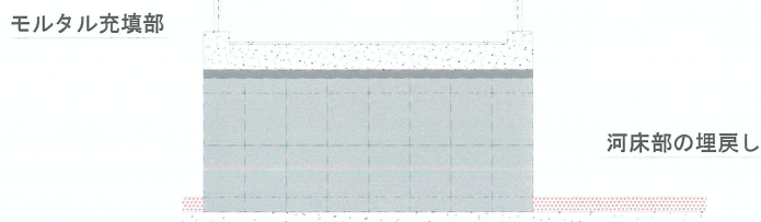
モルタル充填完了 ※上記「施工手順 ⑤」
