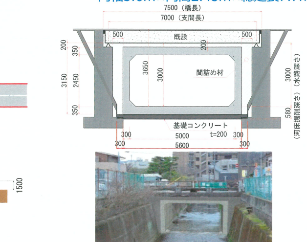
更新（架替え）工事の全体概要図（検討モデル）
