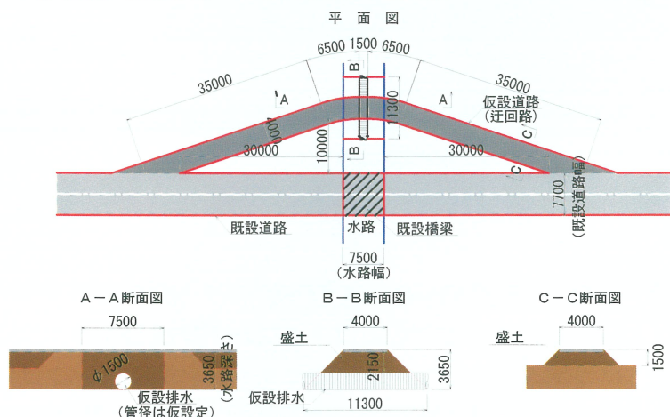
更新（架替え）工事の全体概要図（検討モデル）
