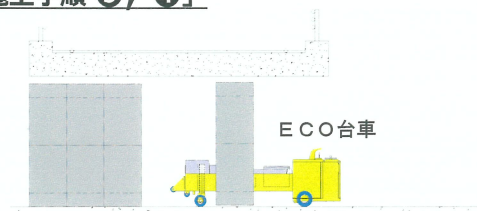
モルタル充填完了 ※上記「施工手順 ⑤」
