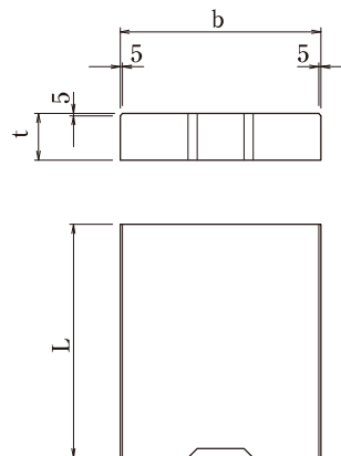
国交省規格蓋(C種)
